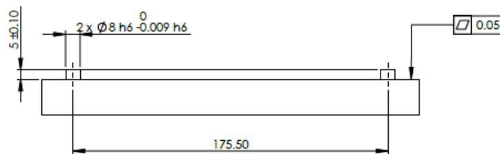
1.2: Montageplatte für Roboterbasis
